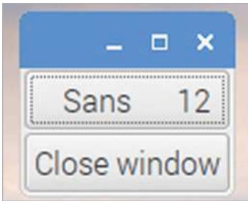
▲ A GtkFontButton
