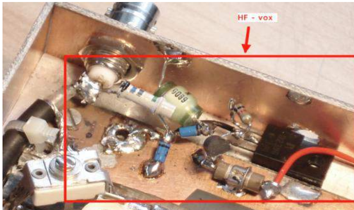
De HF vox-schakeling
