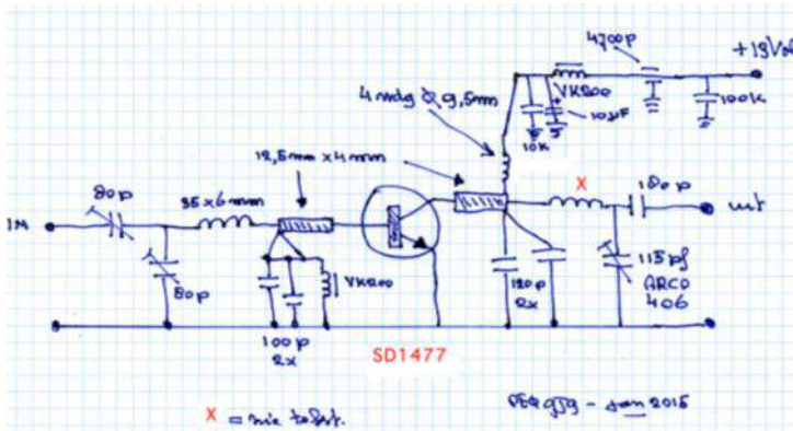
De PEØGJG - SD1477 eindtrap SD1477, januari 2015
